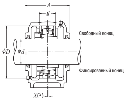
Установочное кольцо
