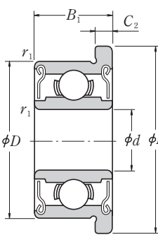
Тип с защитными шайбами ZZ · ZZ1
