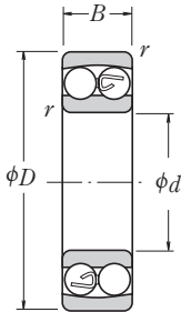
Цилиндрическое отверстие
