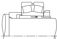
Рис. 14.4. Монтаж с закрепительной втулкой
