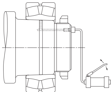
Рис.14.19. Демонтаж с помощью гидронасоса впрыскивающего масла
