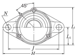
Тип с литой пылезащитной крышкой
