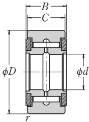
Без сепаратора
