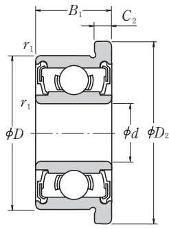
С контактнм уплотнением DD
