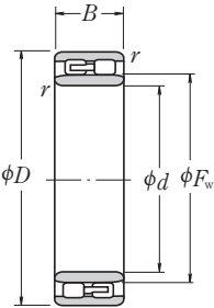
NNU
