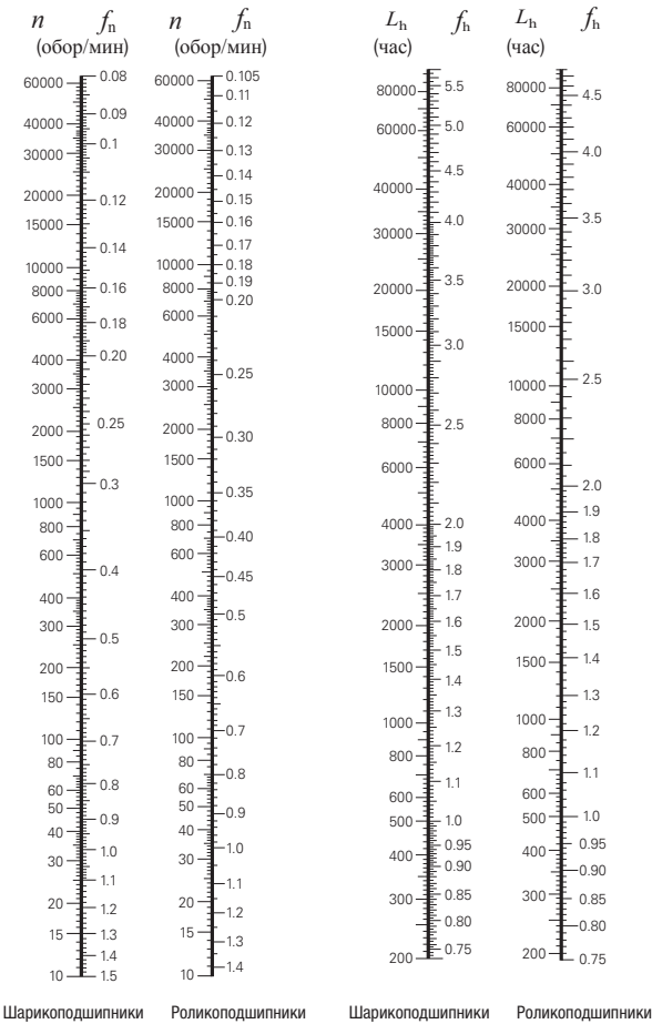
Рисунок 5.3. Скорость вращения подшипника и коэффициент скорости вращения
