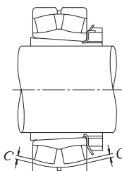
Рис. 14.8. Измерение зазора в сферическом роликоподшипнике
