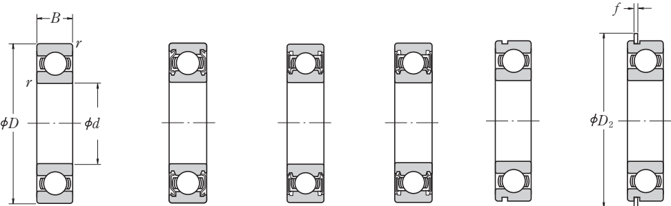
Открытый тип
