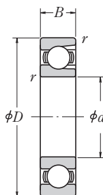
Открытый тип
