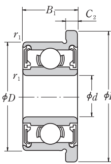
С бесконтактным уплотнением VV
