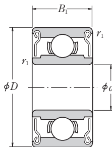
Тип с защитными шайбами ZZ · ZZ1
