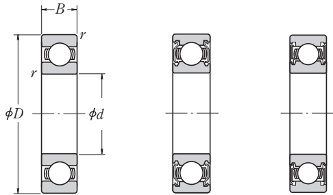
Открытый тип
