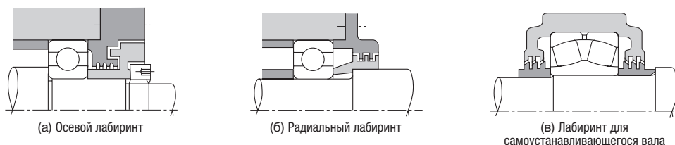
Рис. 11.7. Примеры конструкций лабиринтных уплотнений
