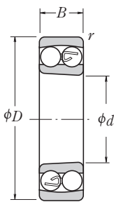
Коническое отверстие
