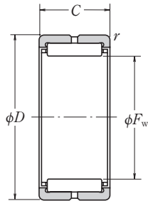
Без внутреннего кольца RNA
