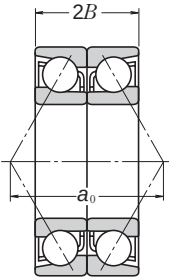
По 0-образной схеме 0B
